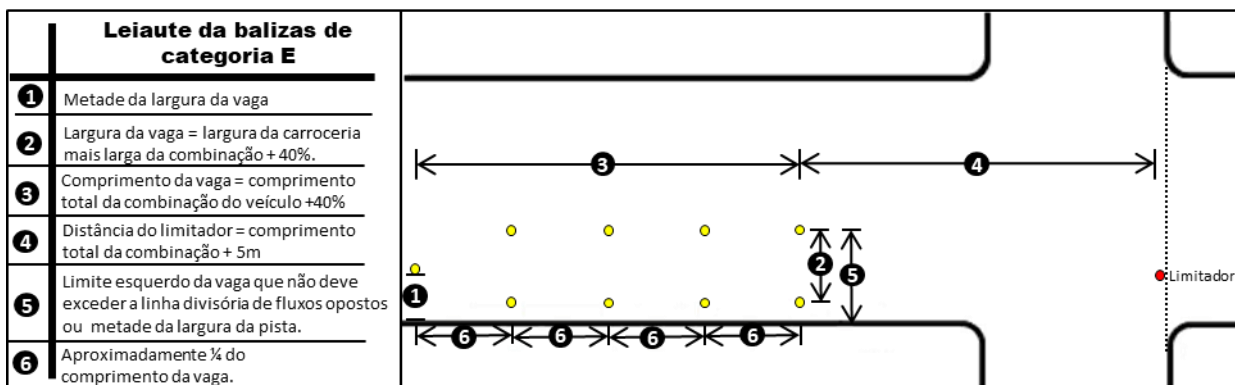
Figura 4: Leiaute de balizas categoria E
