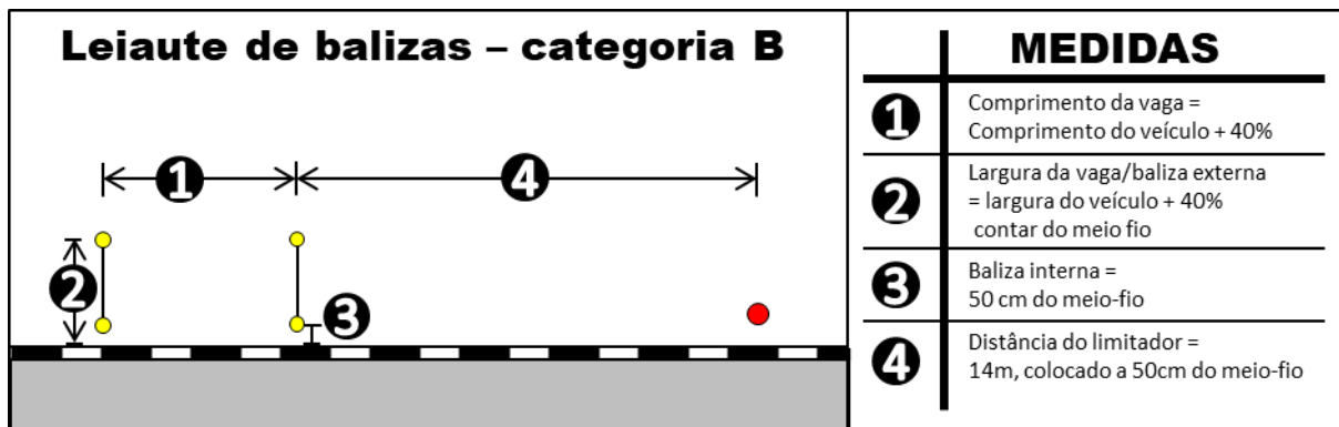
Figura 2: Leiaute de balizas categoria B
