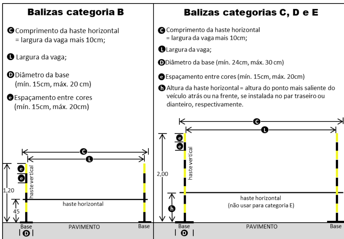
Figura 1: Especificações de balizas
